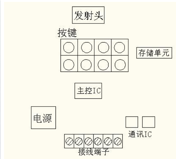
图 2：RS816 遥控器组成
