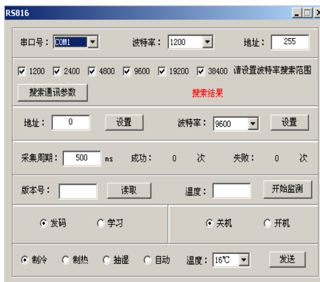
图 6：软件界面
